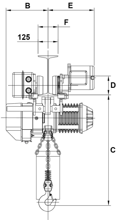
低舉型電動鏈條吊車規格尺寸 / LHR DIMENSIONS (mm)
