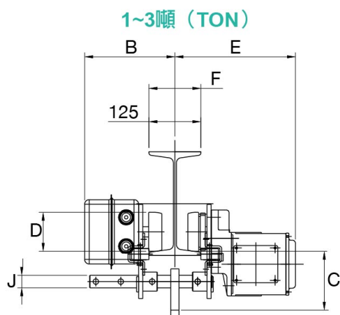
◎ 單軌電動小車規格尺寸 / USM DIMENSIONS (mm)
